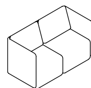
Box2 1360 680 760 / 410
