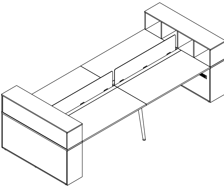
SS45 3700 1540 1100 / 745
